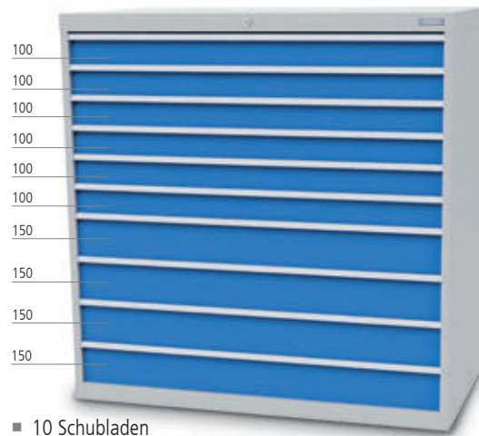
■ 10 Schubladen
