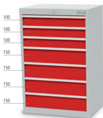
▪ 7 x Schublade
