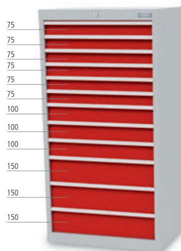
■ 12 x Schublade
