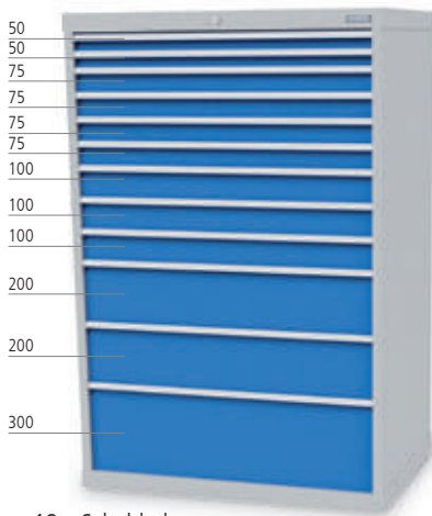
■ 12 x Schublade
