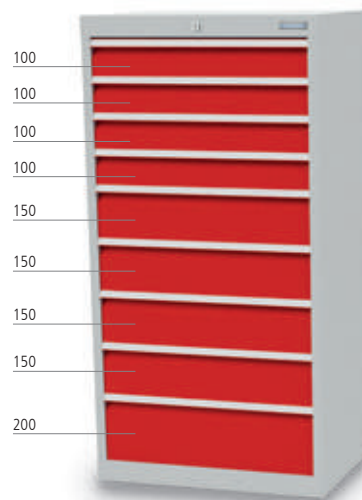
■ 9 x Schublade
