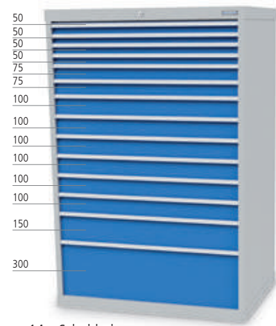
■ 14 x Schublade
